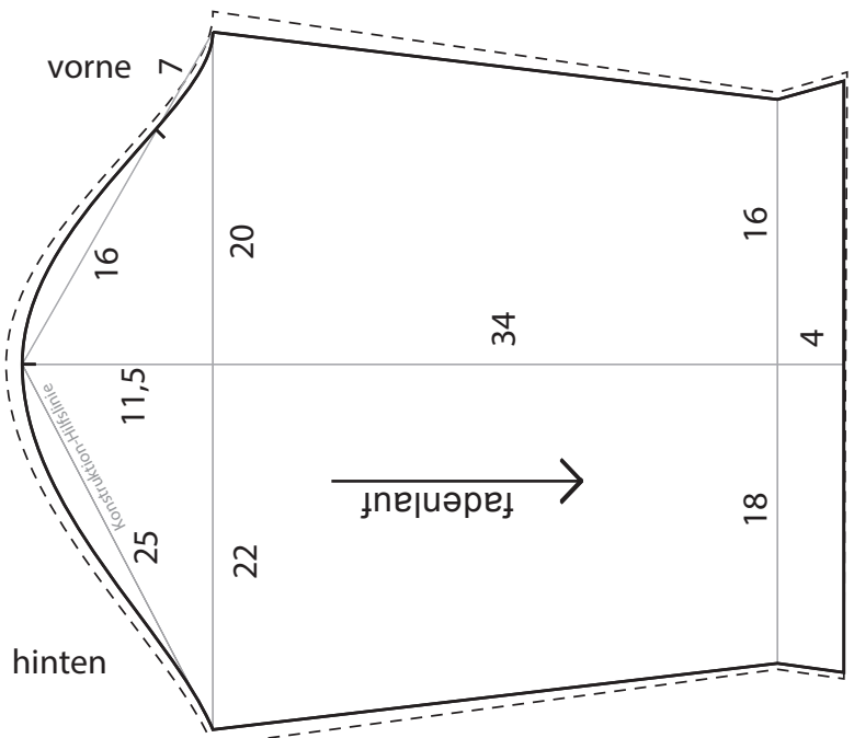
Ärmel 1cm Nahtzugabe enthalten 4cm Saum enthalten
