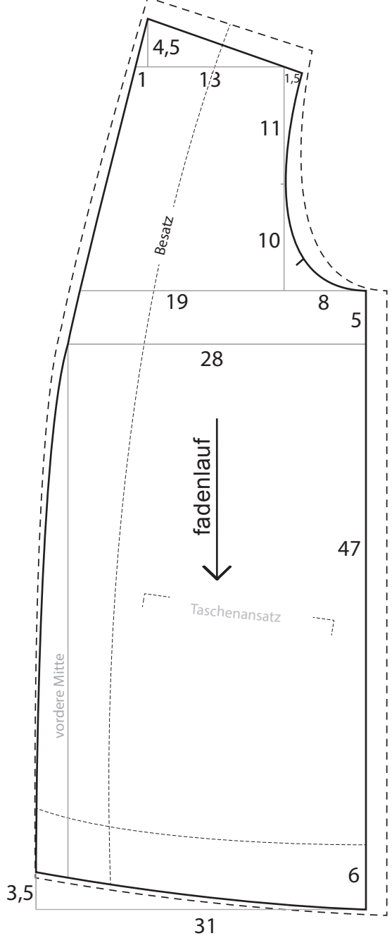
Vorderteil 1cm Nahtzugabe enthalten 6cm Saum
