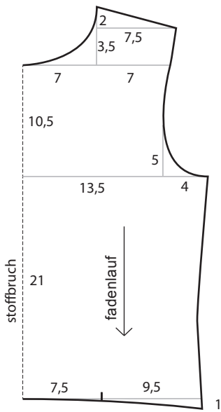
Vorderteil 1 cm Nahtzugabe enthalten
