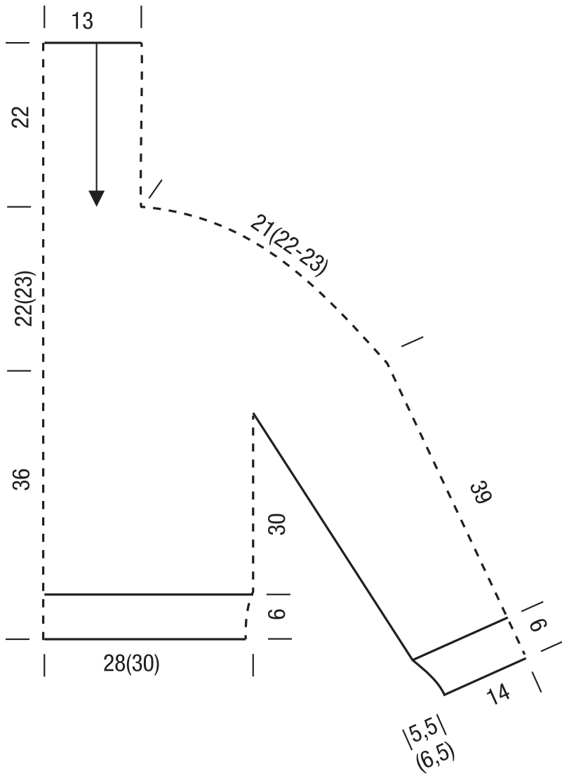
Rücken- und Vorderteil Hälfte
