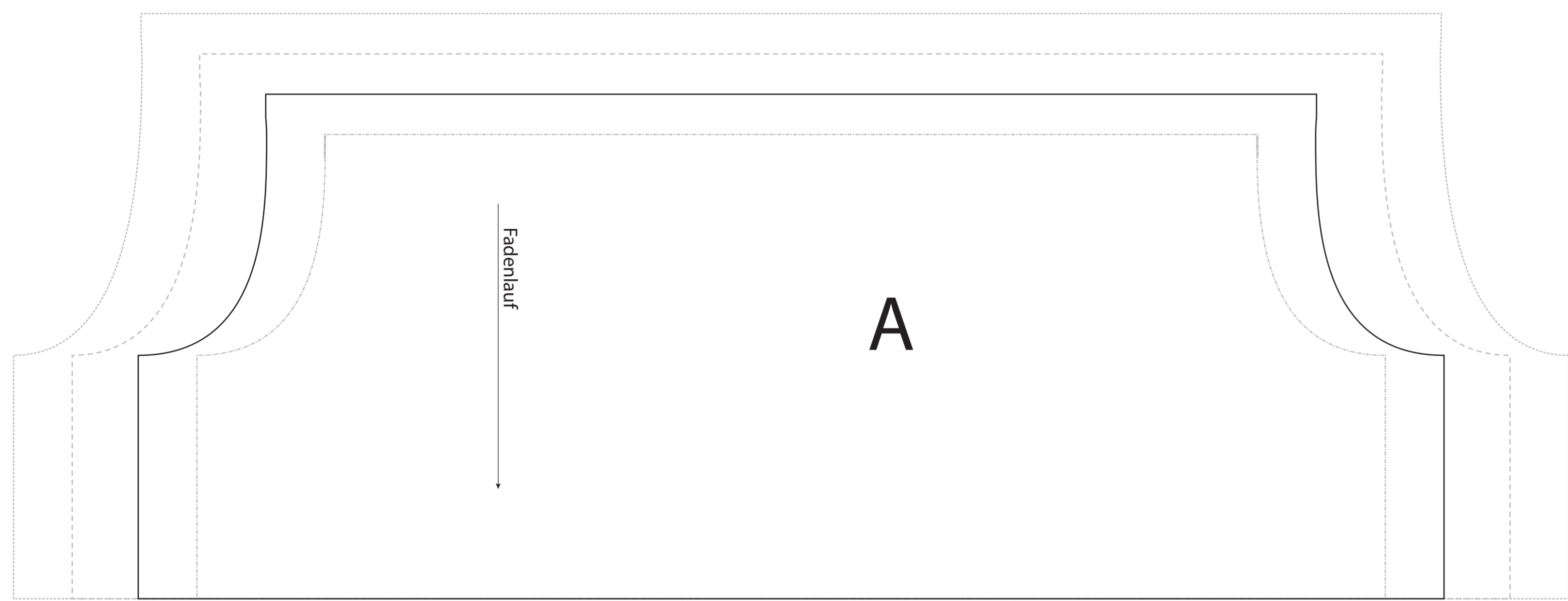
oberes Vorderteil
