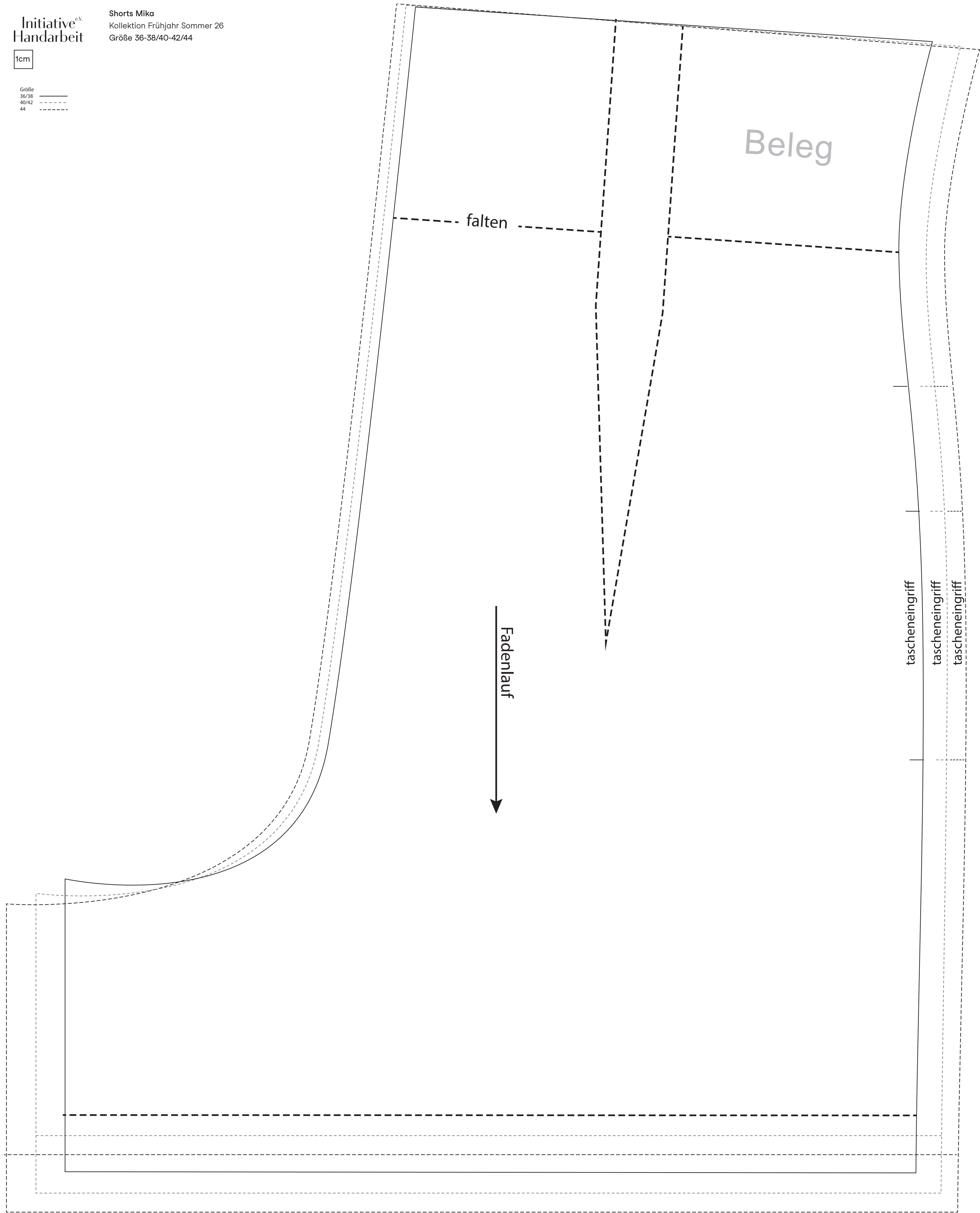
Rückw. Hosenteil
