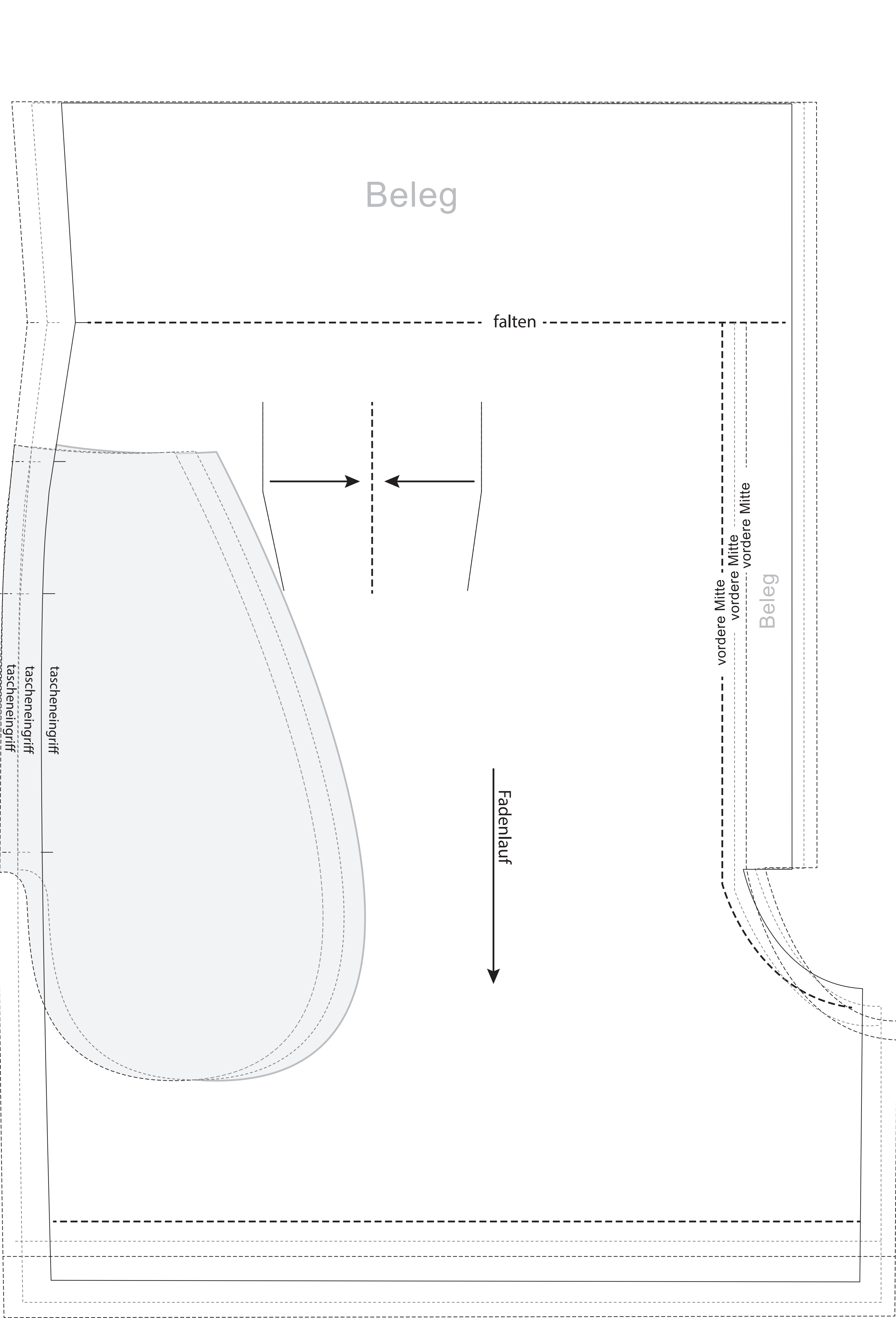
Vord. Hosenteil
