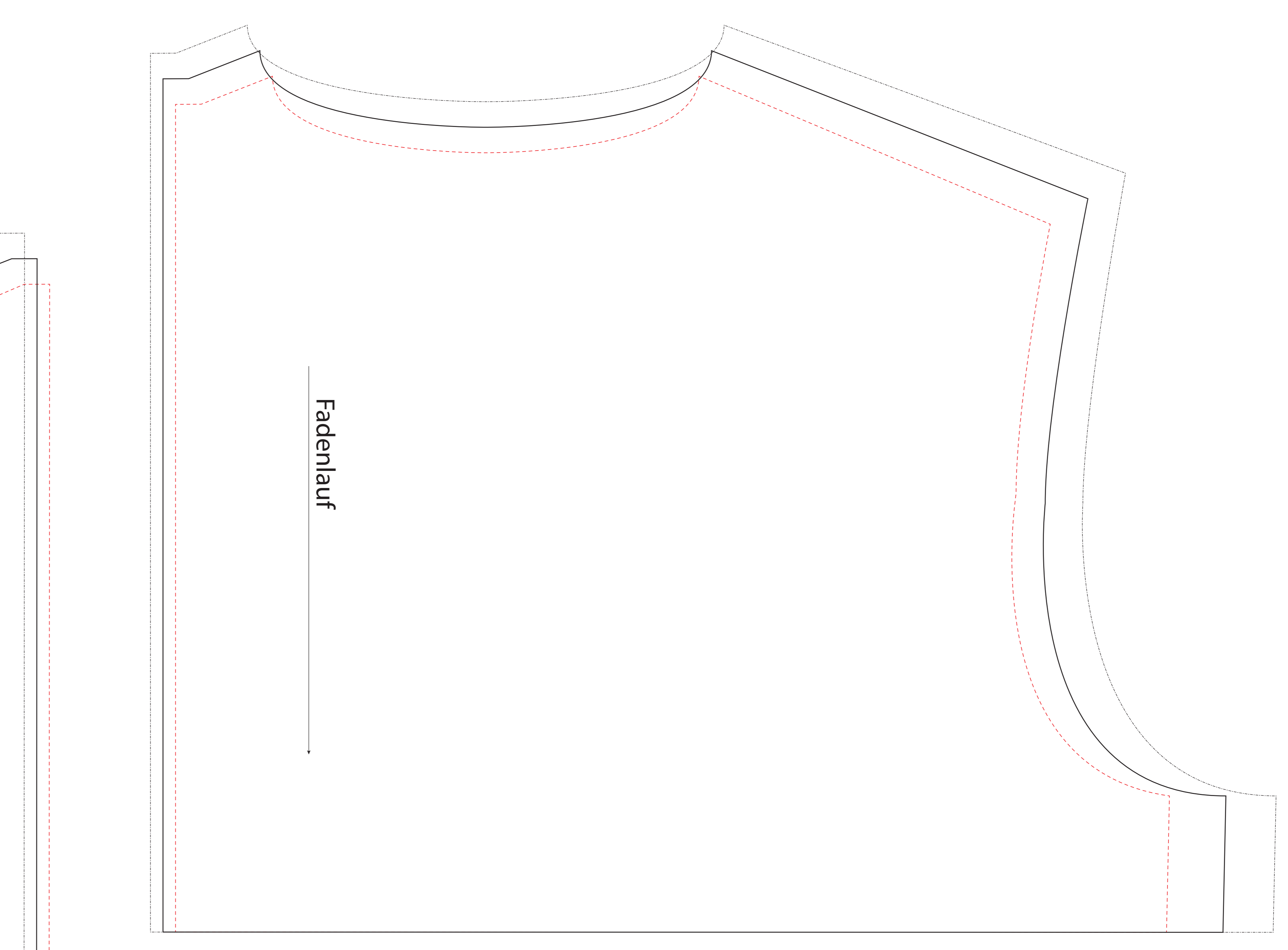
Rückenteil A
