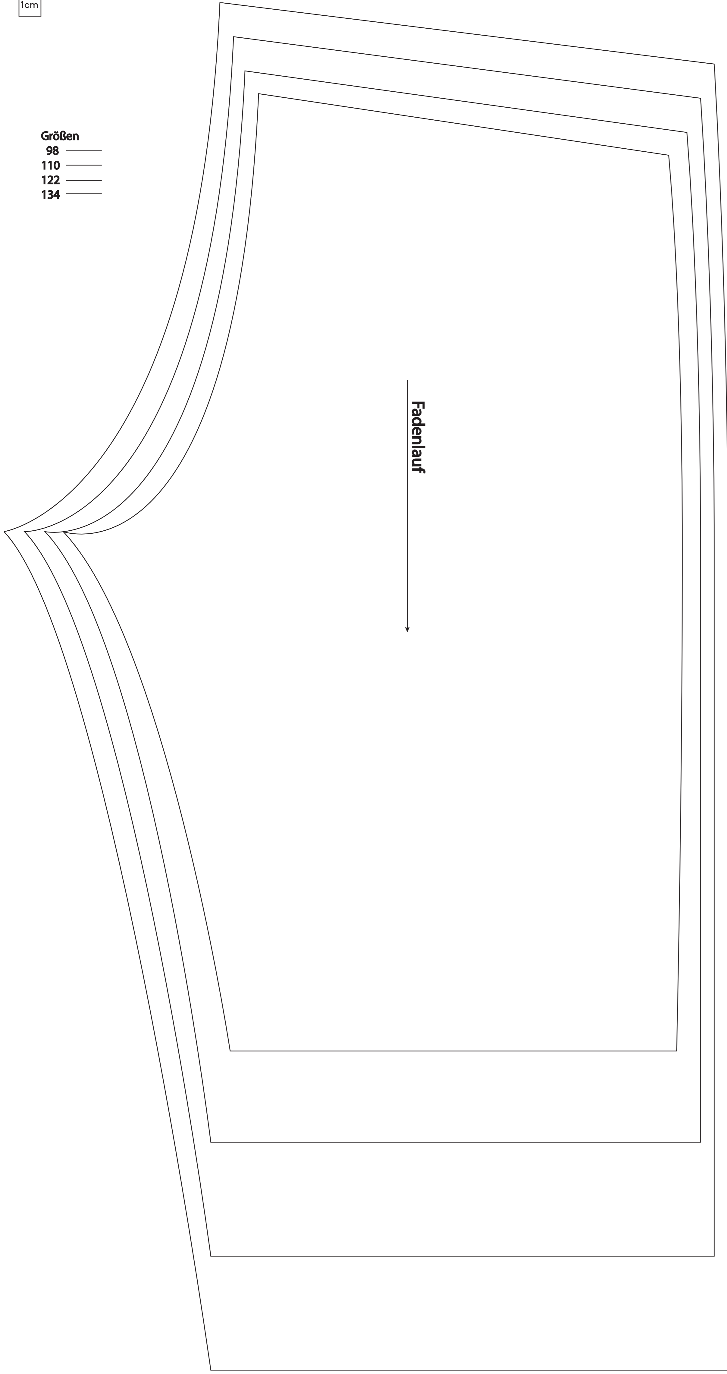
Hinteres Hosenteil
