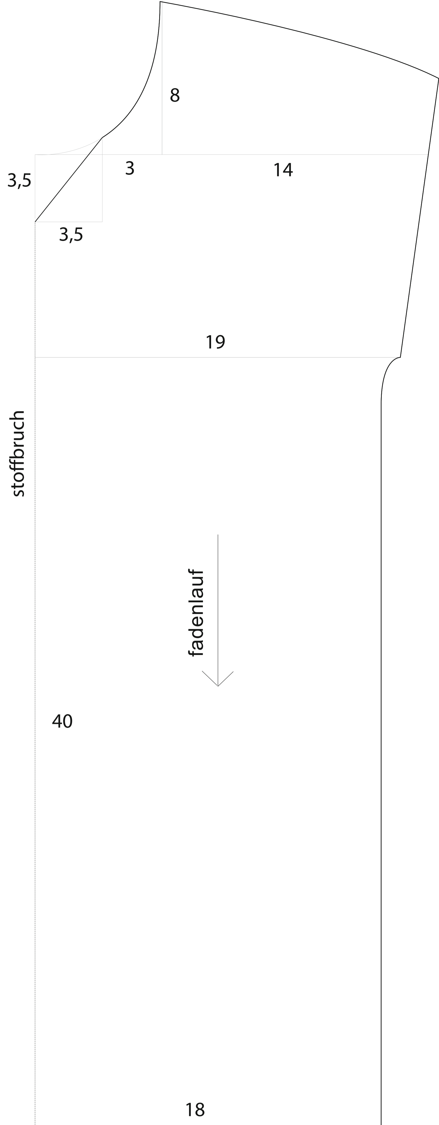
Vorderteil 0,6 cm Nz enthalten
