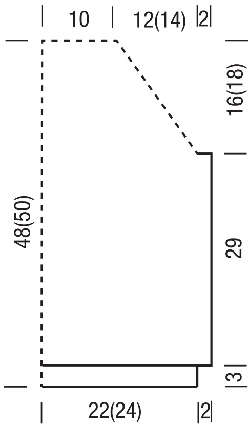
Rücken- und Vorderteil Hälfte
