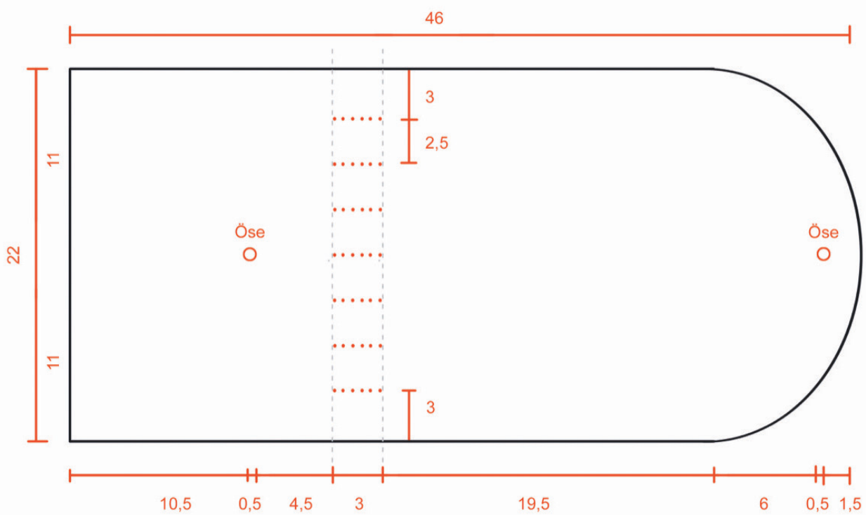
Buch für DIN A 4, alle Abmessungen in cm
