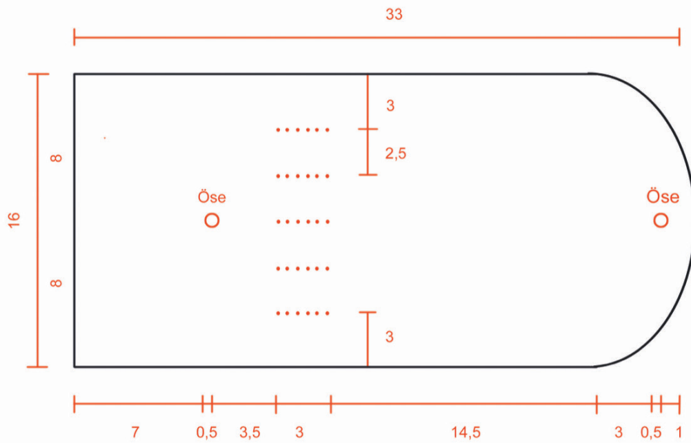
Buch für DIN A 5, Abmessungen in cm
