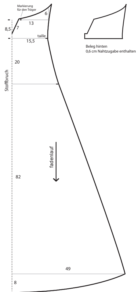
Rückenteil 0,6 cm Nahtzugabe enthalten 1,5 cm Saum enthalten
