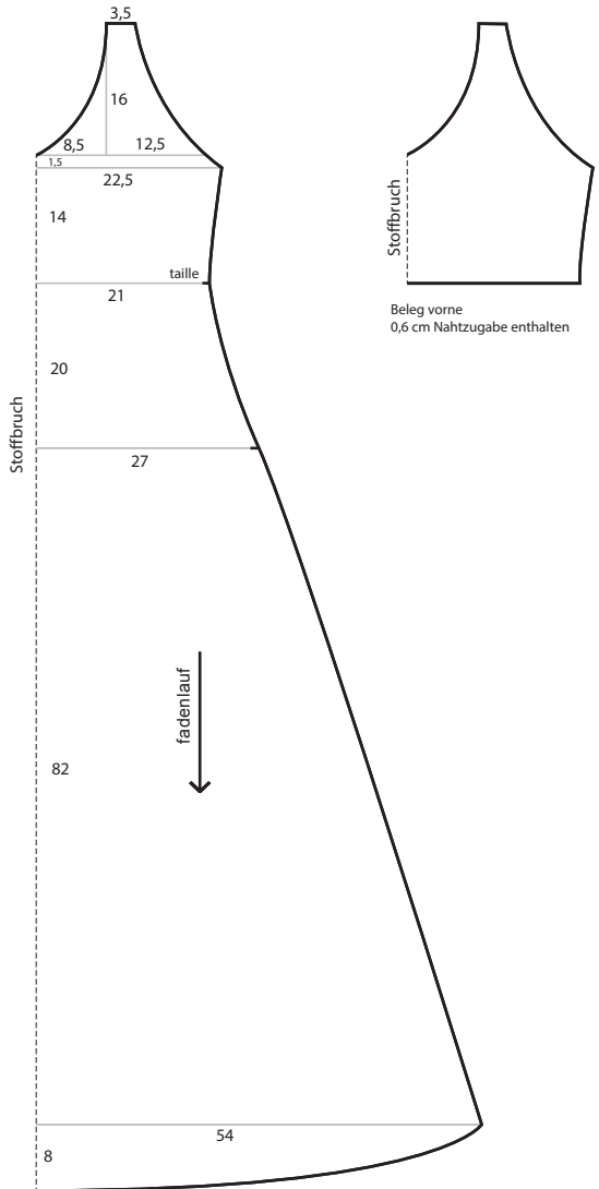
Vorderteil 0,6 cm Nahtzugabe enthalten 1,5 cm Saum enthalten
