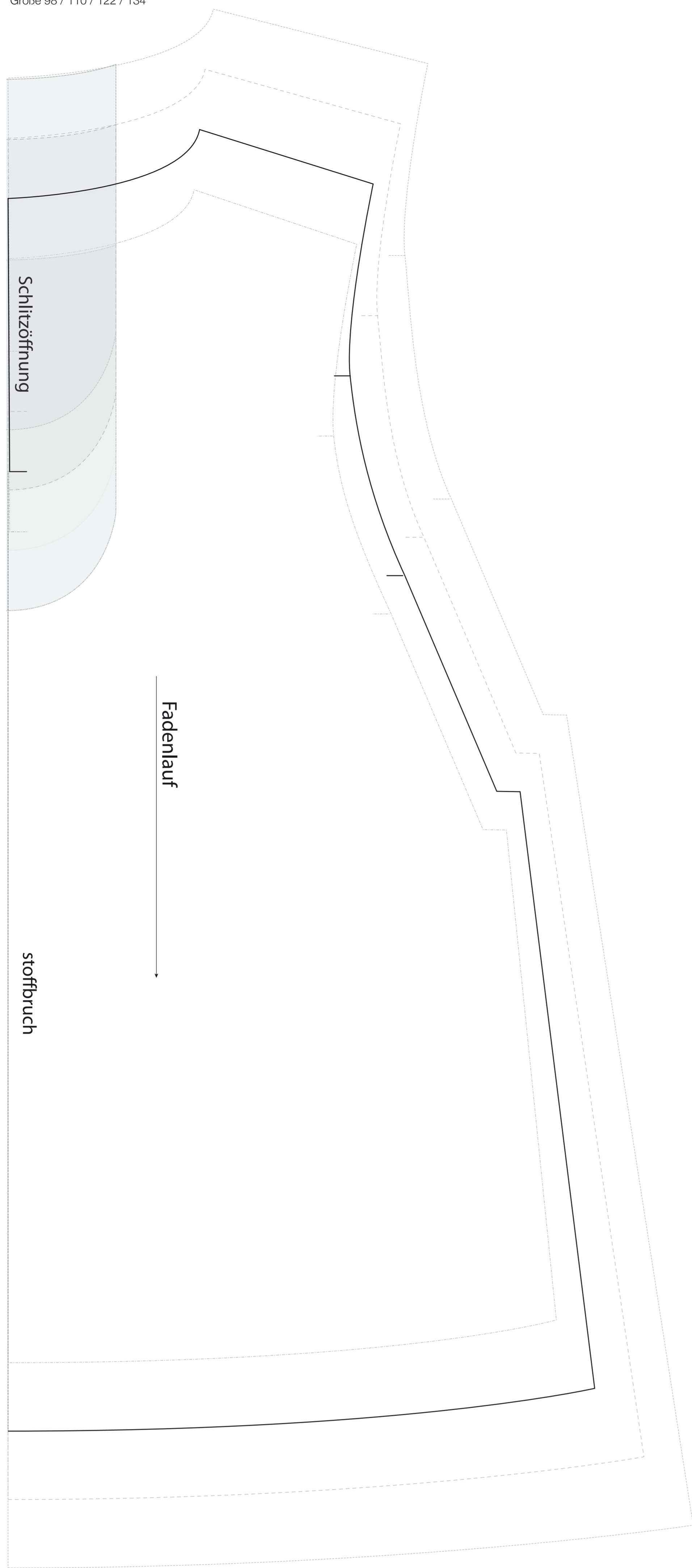
Rückenteil
