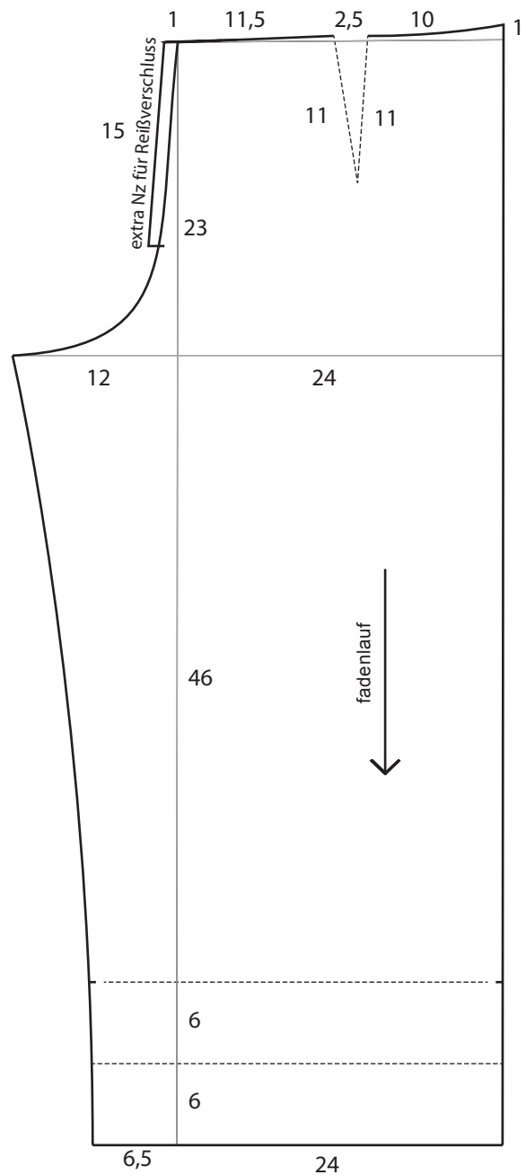
Hinteres Hosenteil 1cm Nahtzugabe und Saum enthalten
