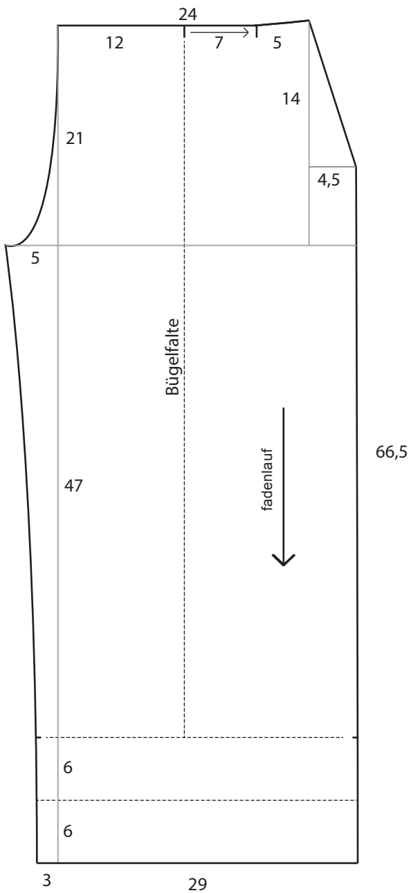
Vorderes Hosenteil 1cm Nahtzugabe und Saum enthalten
